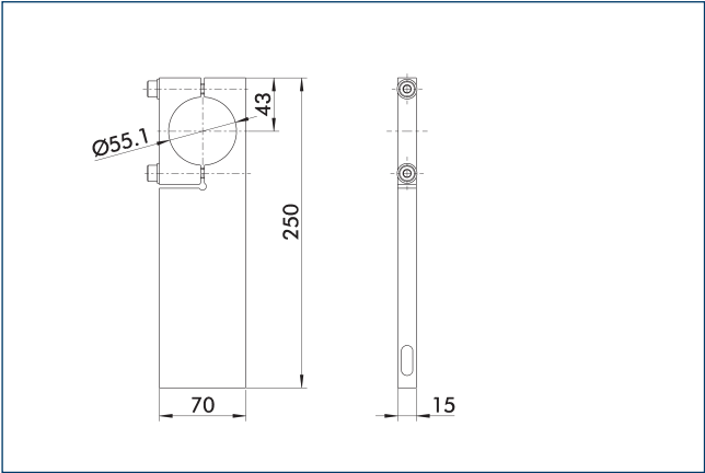
用于延伸和支撑立柱装配系统的安装板
