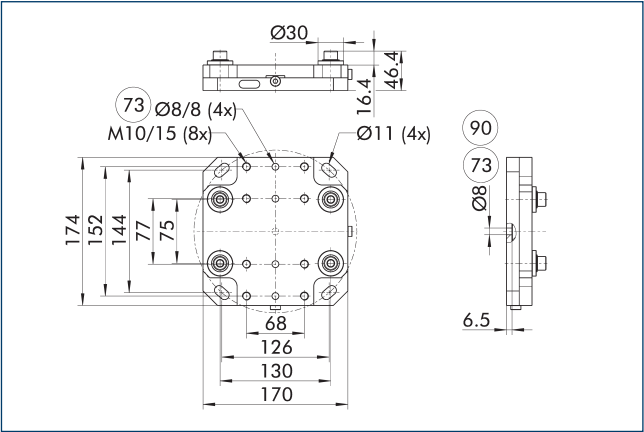
73 适合定心销 90 定中作为旋转的轴
