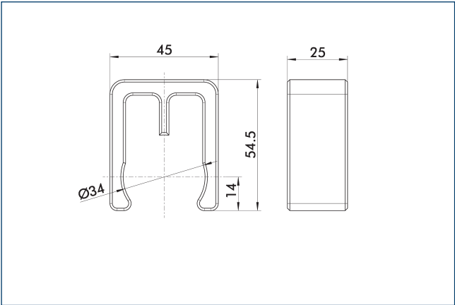
用于沿支柱整齐布置介质管路的固定夹。
